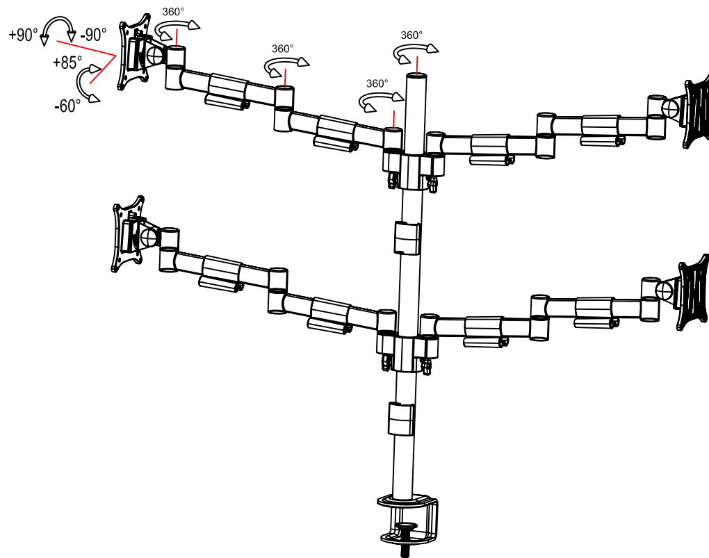
多功能调节示意图
